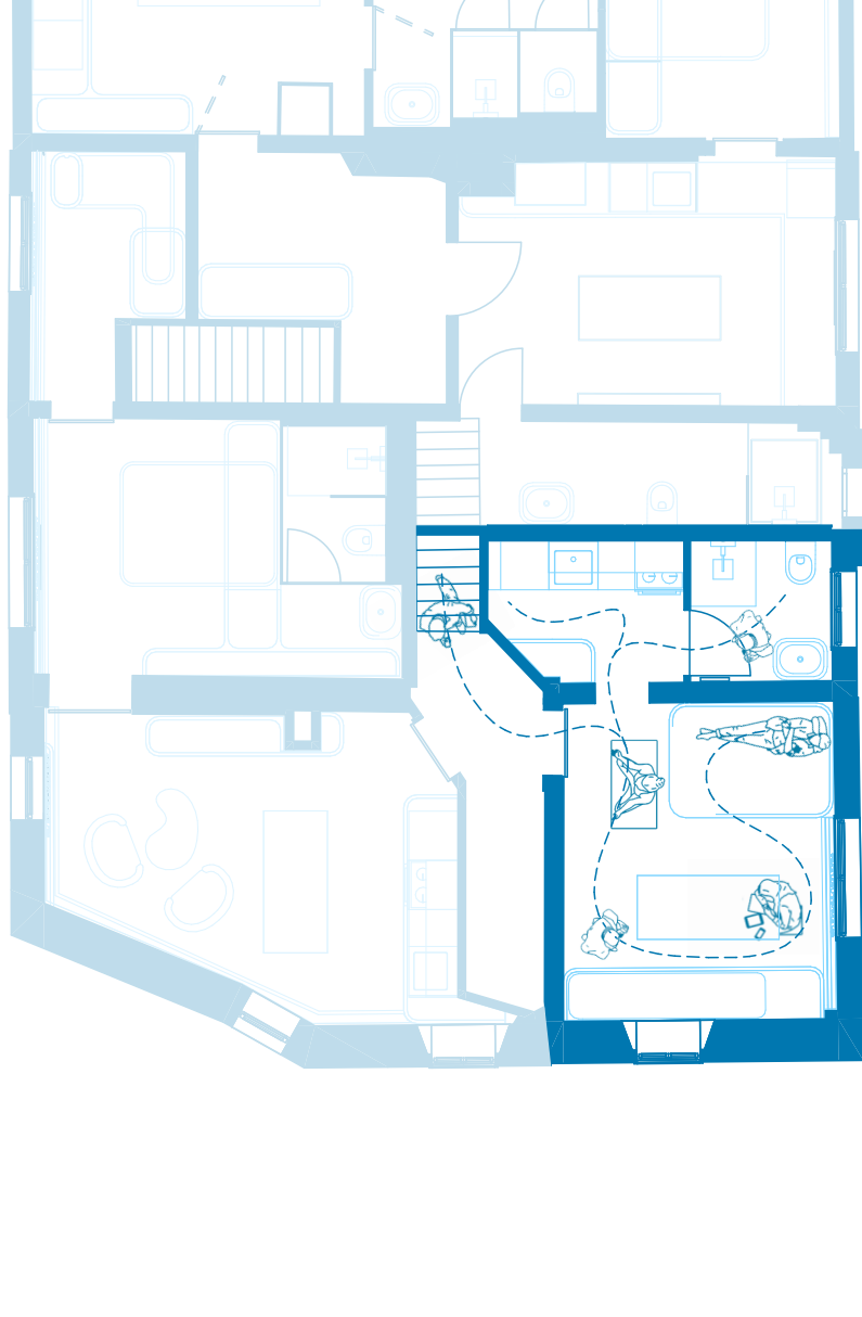
wohnung 5 20.00 m² 1:100
