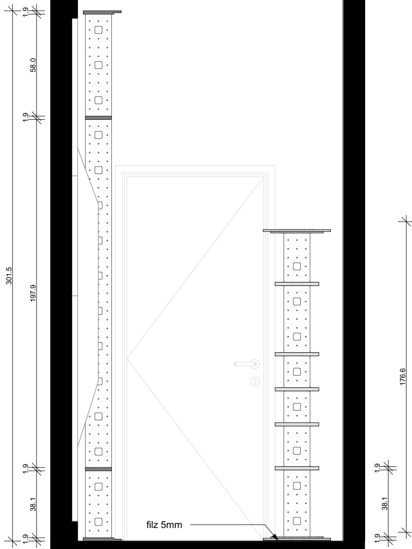
section d-d
